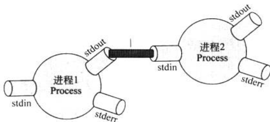
图 7.2 用于连接两个进程的管道
