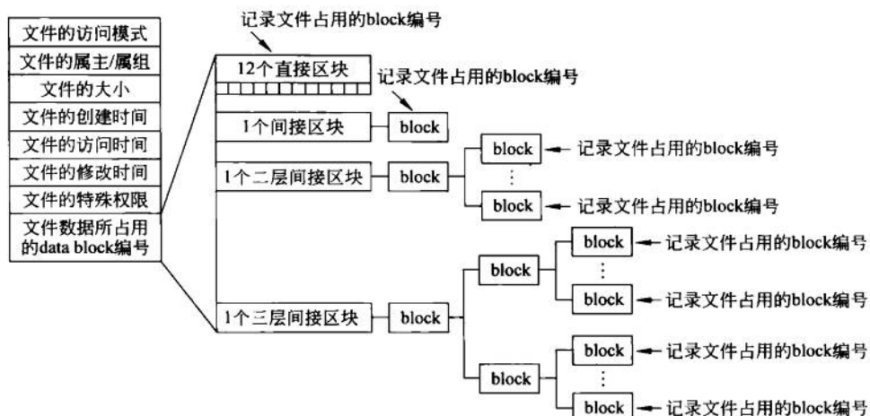
图 9.5 inode 的分层式结构
