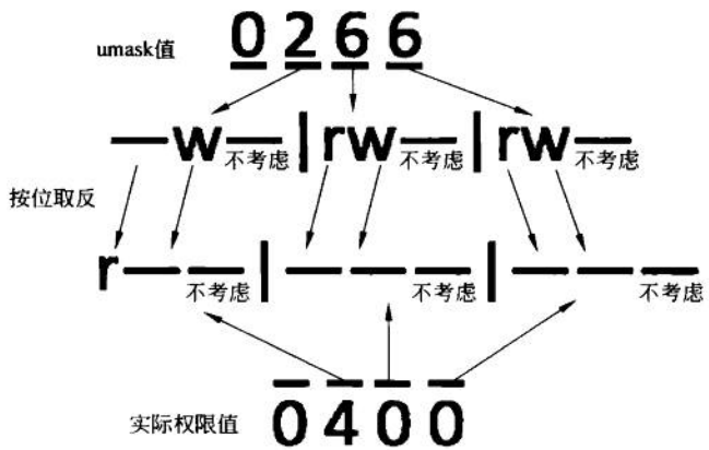
图 6.5 umask 值与实际权限值
