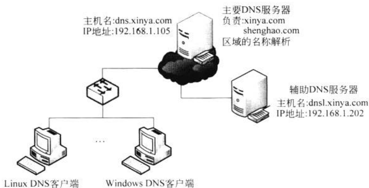
图 22.6 BIND 服务器构建模型
