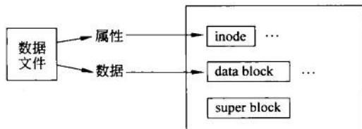
图 9.2 文件的分开存储
