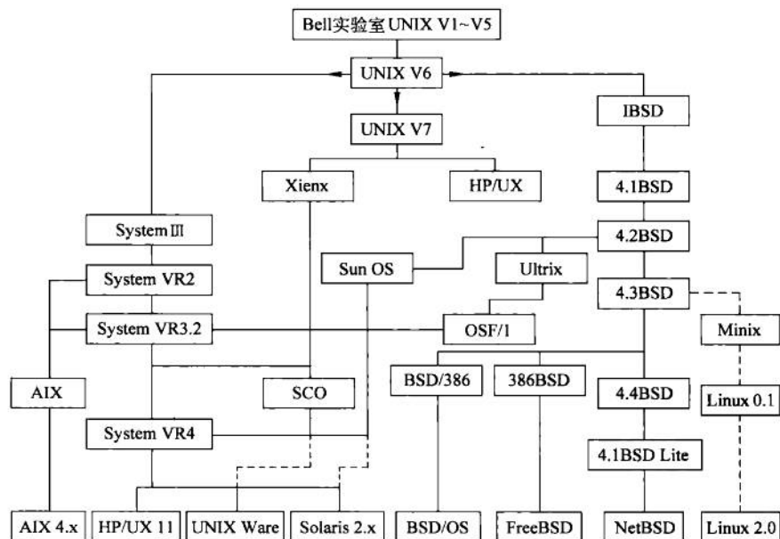
图 1.4 UNIX 发展路线图
