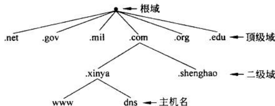
图 22.1 域名空间结构图
