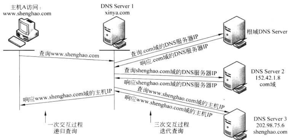
图 22.4 DNS 服务器的查询过程
