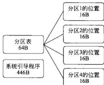
图 2.6 DPT 的结构
