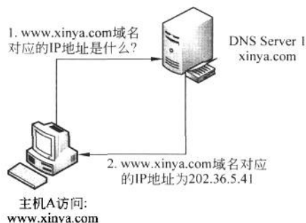
图 22.2 本区域的 DNS 查询过程
