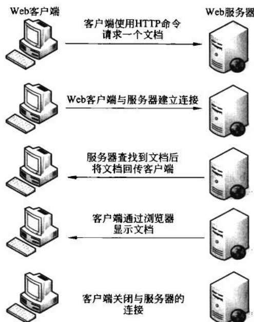
图 23.1 HTTP 协议的通信过程
