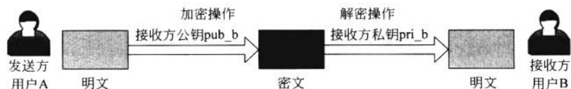
图 24.4 非对称加密
