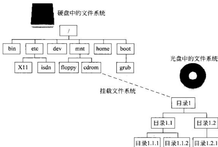
图 10.1 挂载文件系统
