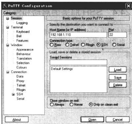
图 24.1 PuTTY 的配置界面
