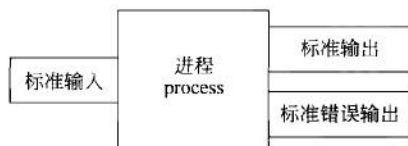
图 7.1 进程的标准通道
