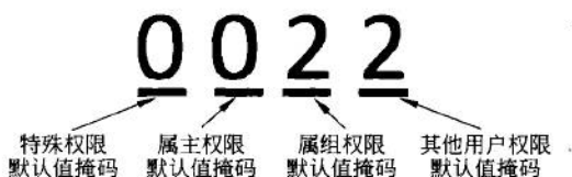
图 6.2 umask 掩码的结构
