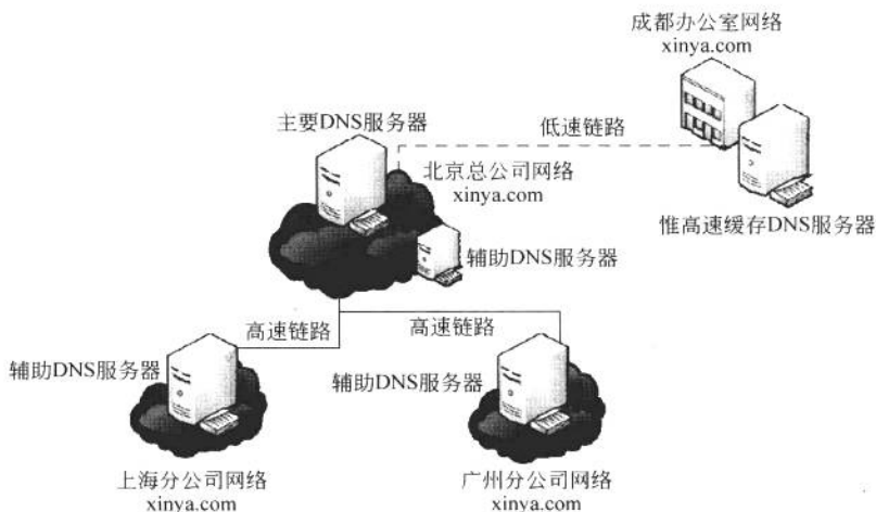
图 22.5 DNS 服务器的种类
