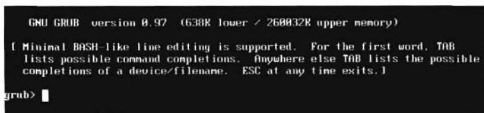
图 15.4 GRUB 的命令行界面
