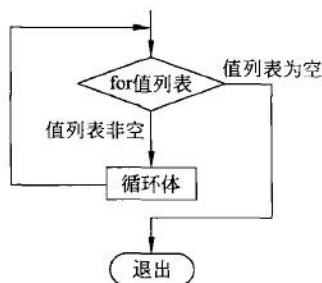
图 19.4 for 语句的语法结构图
