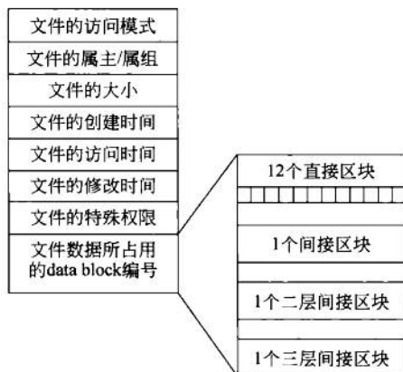
图 9.4 inode 中的 data block 记录结构
