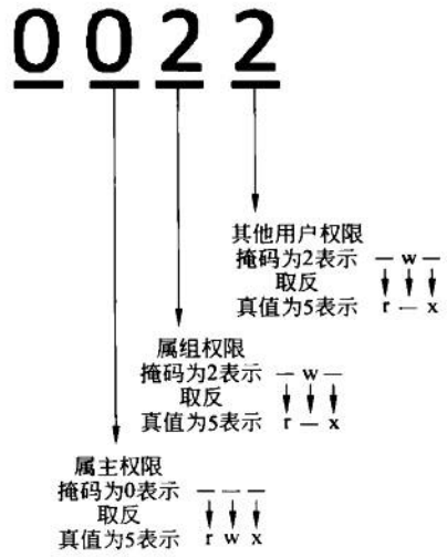
图 6.4 目录的默认权限掩码
