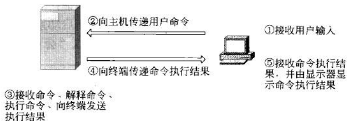
图 3.2 主机-终端的工作模式
