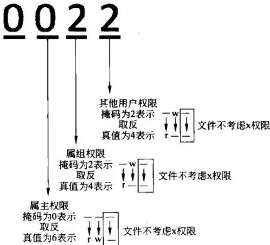
图 6.3 文件的默认权限掩码
