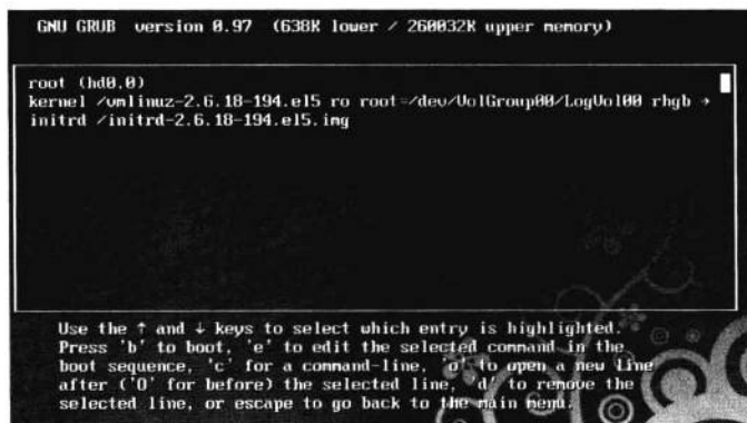
图 15.3 GRUB 的启动菜单项编辑界面
