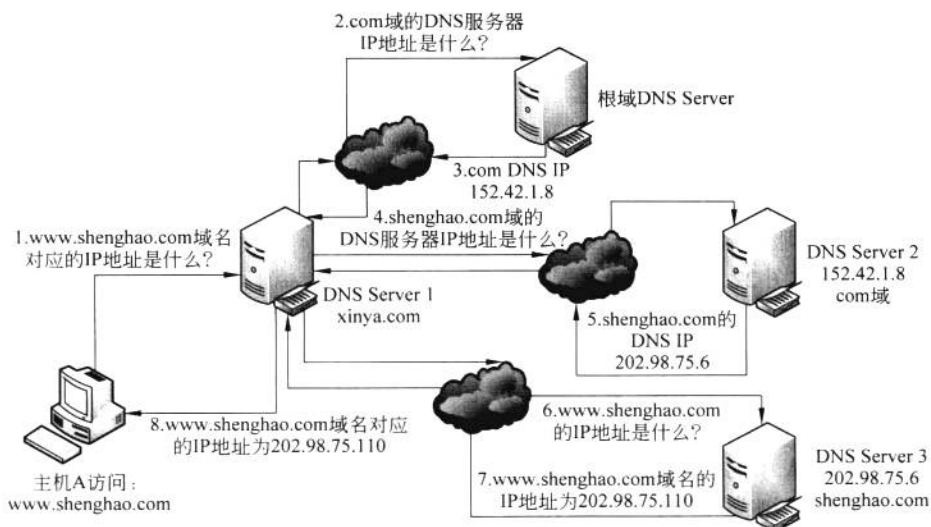
图 22.3 DNS 查询过程
